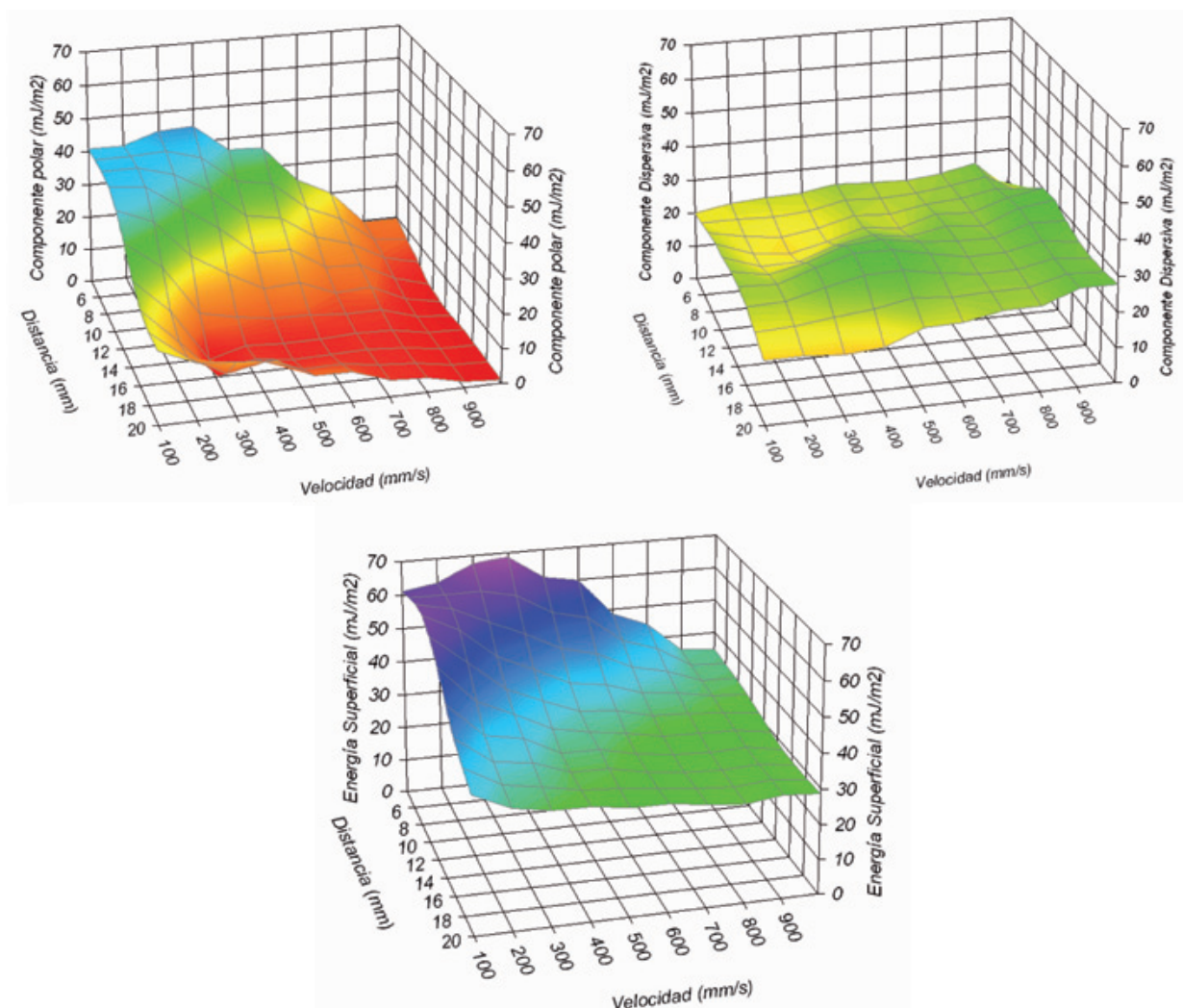
Fig. 3: Representación de la componente polar (superior izquierda) y dispersiva (superior derecha) vista en perspectiva 3D. Abajo representación de la energía superficial total.
