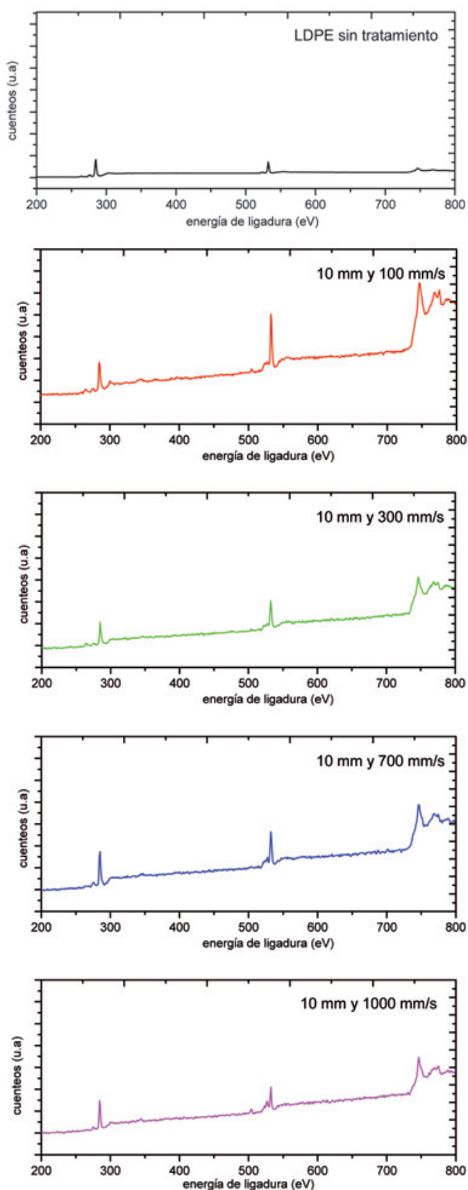
Fig. 5: Espectro XPS de baja resolución de una muestra sin tratar y de muestras tratadas a una distancia de 6 mm y diferentes velocidades
