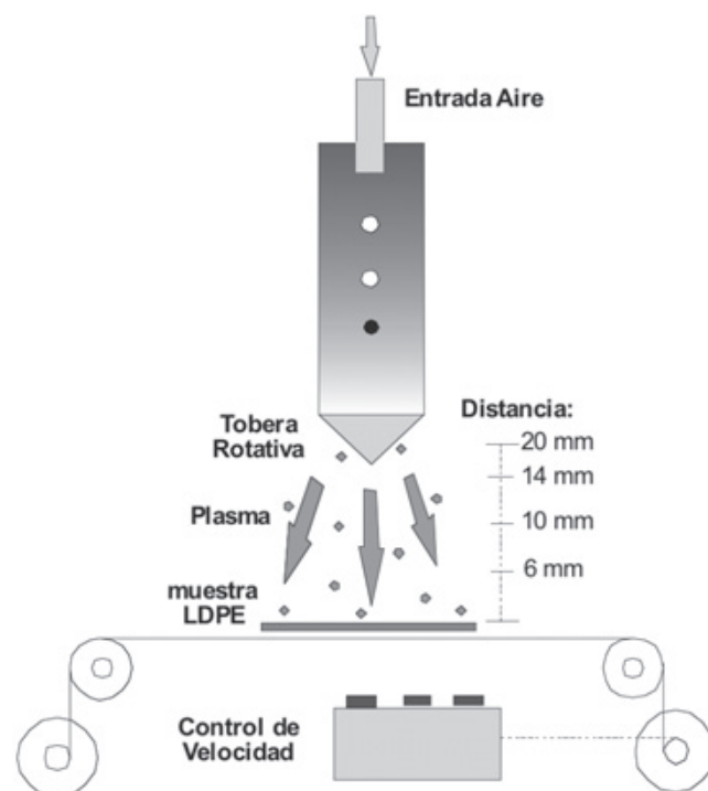
Fig. 1: Esquema de funcionamiento de tratamiento de plasma atmosférico
