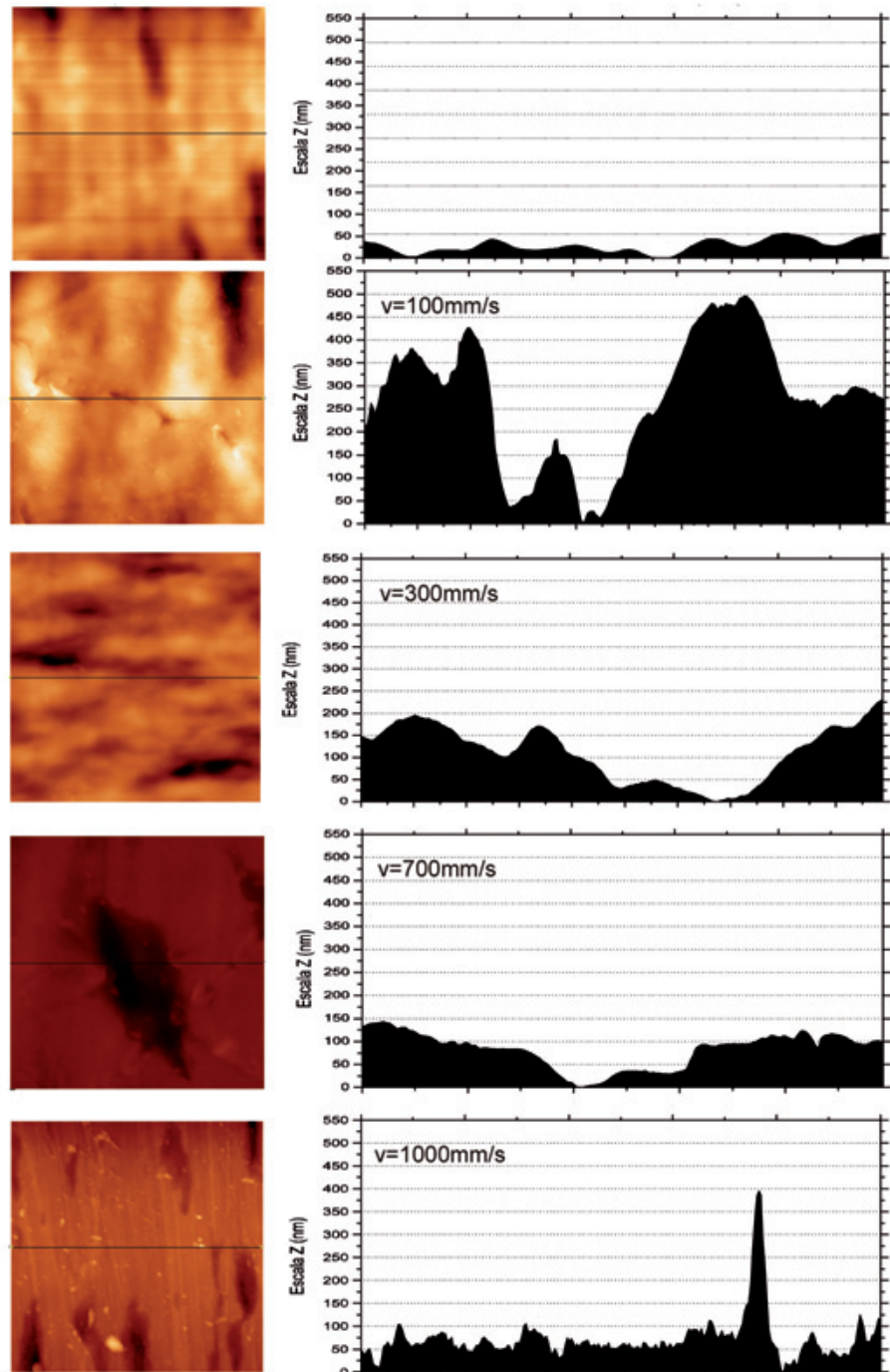
Fig. 4: Perfil de rugosidades de una muestra sin tratar y muestras tratadas a diferentes velocidades a 6 mm de distancia.
