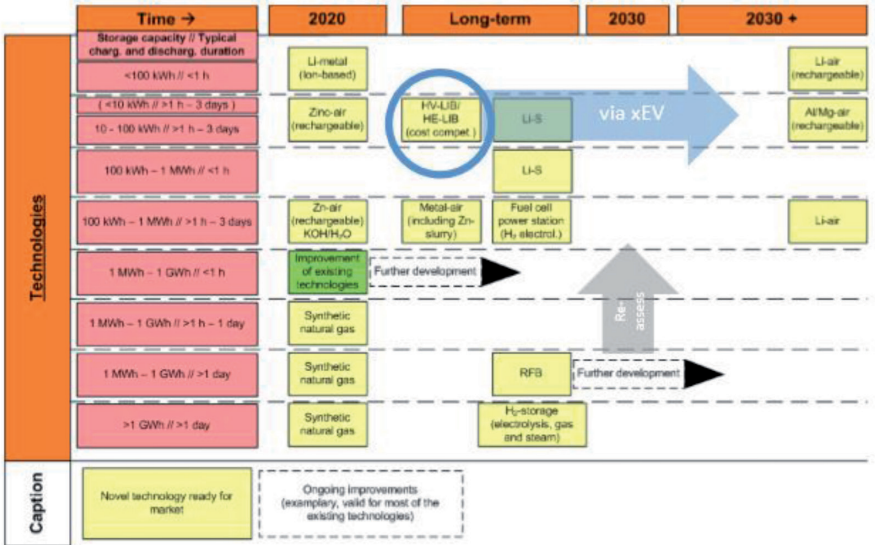
Figura 2: Futuras tendencias en baterías para aplicaciones estacionarias [6]
