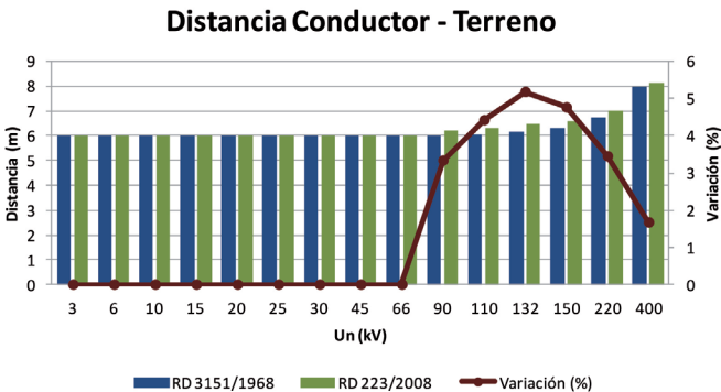
Fig. 3: Distancias de seguridad conductor-terreno según ambos reglamentos
