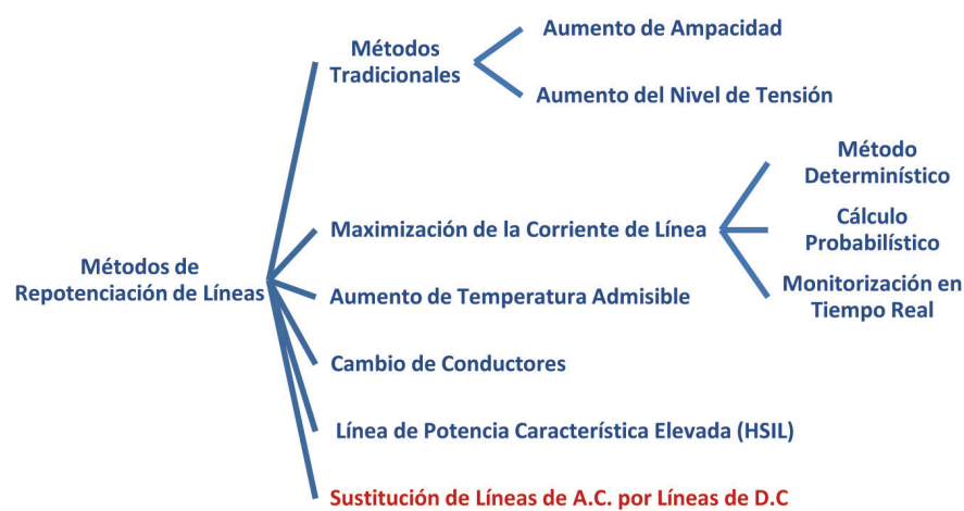
Fig. 1: Alternativas en la repotenciación de líneas eléctricas
