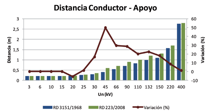
Fig. 5: Distancias de seguridad conductor-apoyo según ambos reglamentos
